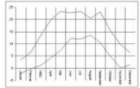
Temperaturverlauf
