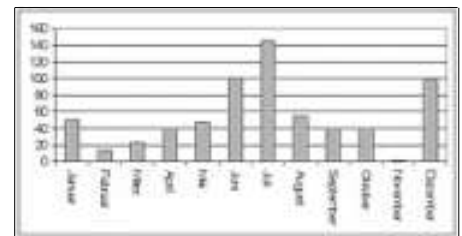
Niederschlagsverteilung
